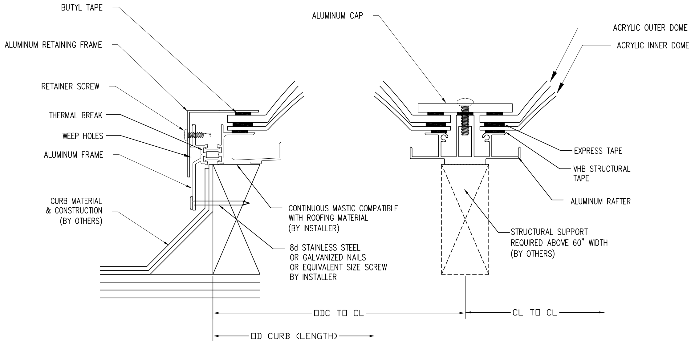
1 SILL SECTION SCALE: 6" = 1'
